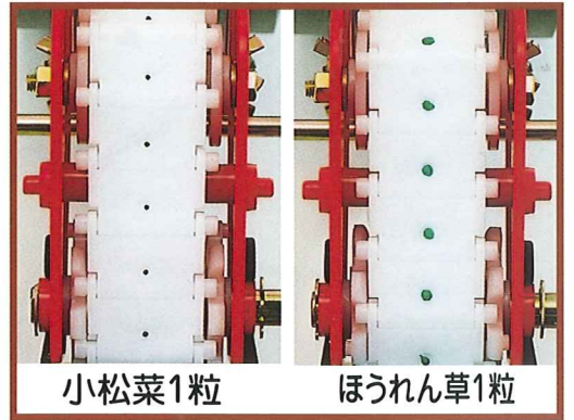
播種ピッチ変更部
