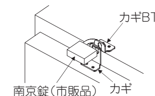
南京錠取付金具詳細
