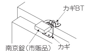
南京錠取付金具詳細
